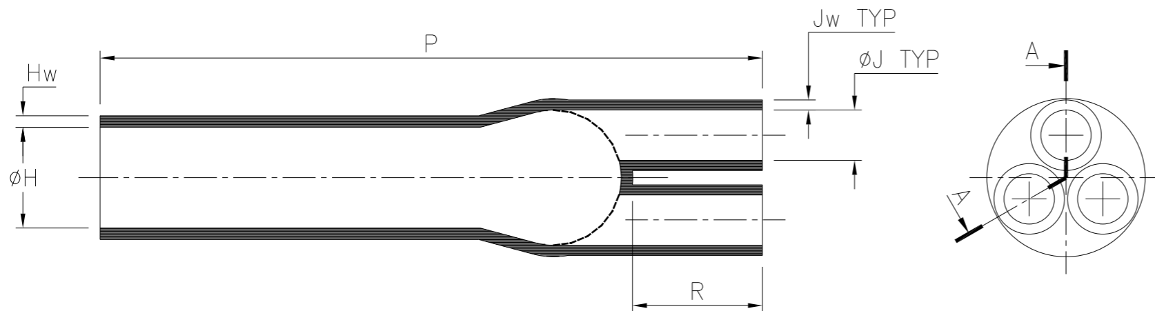
SECTION A-A
